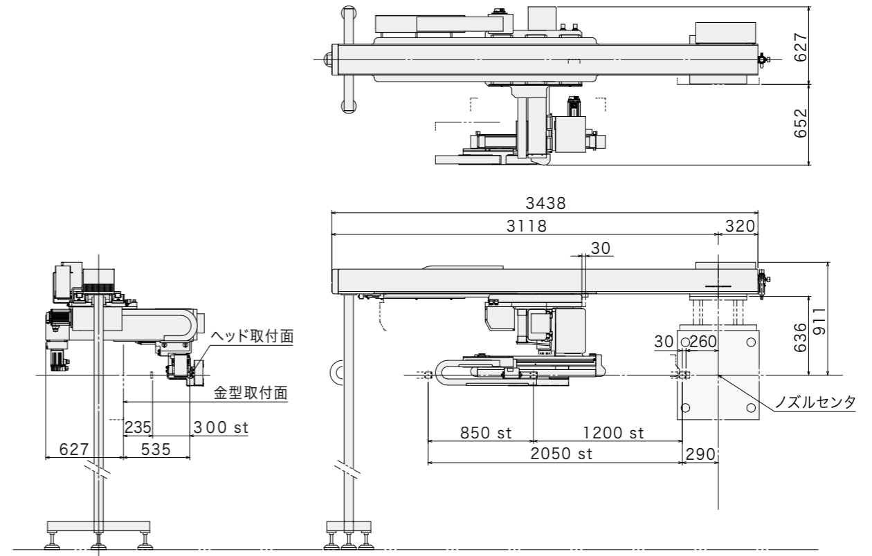
外形寸法図 [mm]
