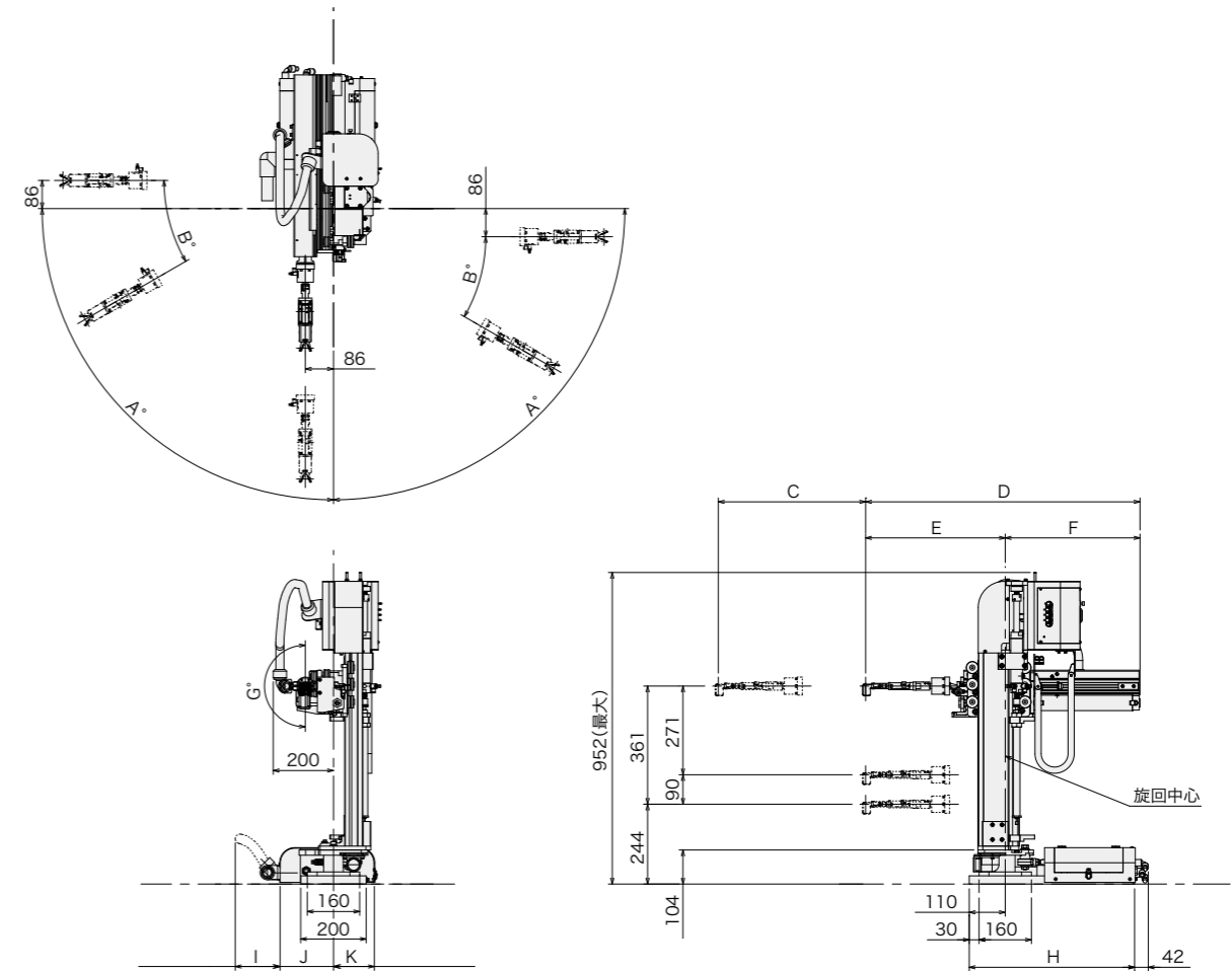
外形寸法図 [mm]
