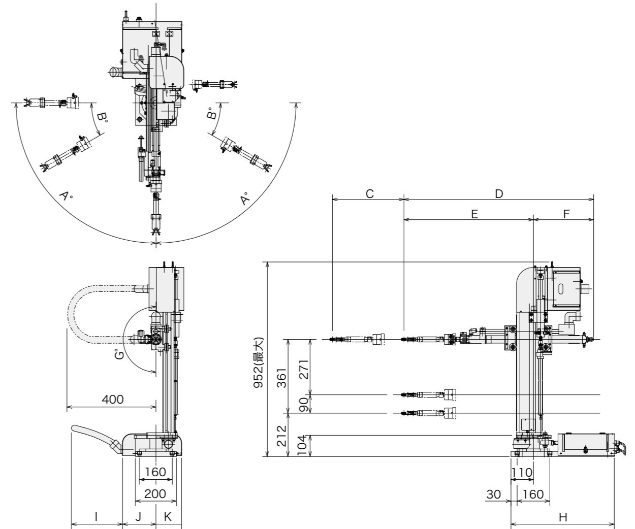
外形寸法図 [mm]
